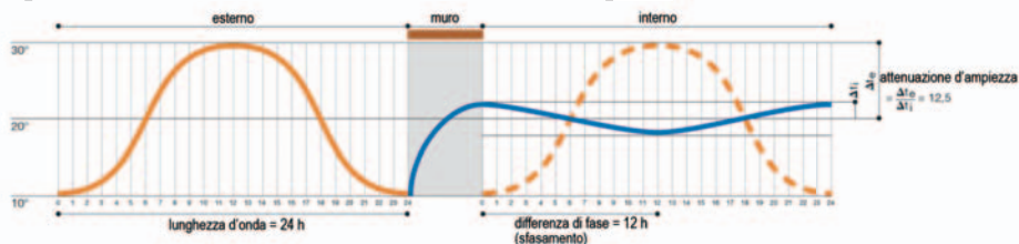
Figura 1 – Sfasamento ed attenuazione dell'onda termica.
