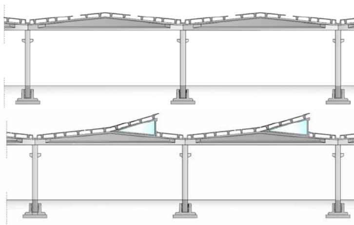
Figura 1. Copertura a doppia pendenza con elementi nervati
